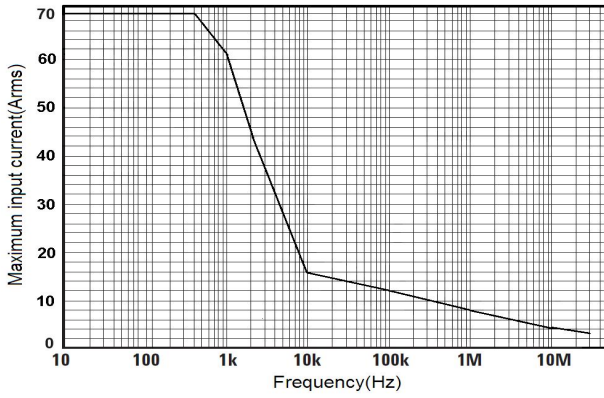
图 8 HCP8070 最大测量电流 VS 频率曲线
